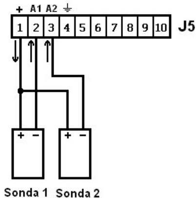
Conexión sondas 4-20 mA 2 hilos alimentadas por el TAF+ (pasivas)
