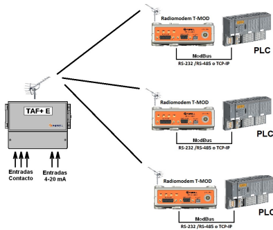
b) TAF E + n x ( T-MOD + PLC )
