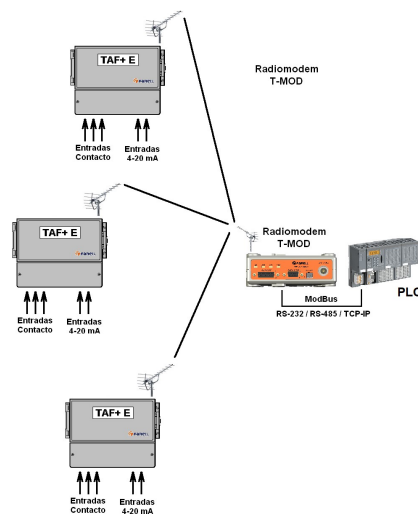
a) n x TAF E + ( T-MOD + PLC )
