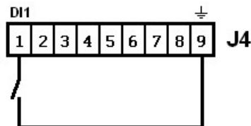
Entrada digital 1 (por contacto)
