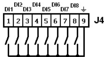
Entradas digitales 1 a 8 ( por contacto )
