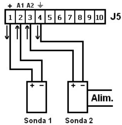
Conexión sondas 4-20 mA Sonda 1 pasiva y sonda 2 activa
