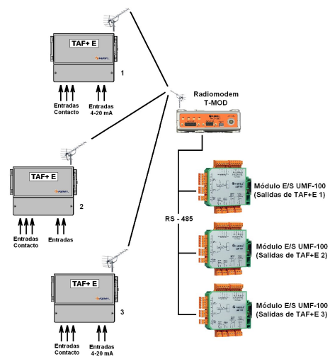
b) n x TAF E + ( T-MOD + n x UMF-100 )
