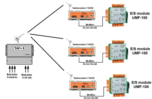
c) TAF E + n x ( T-MOD + UMF-100 )
