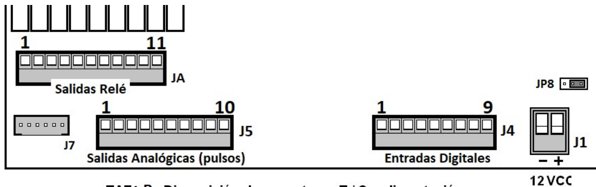
TAF+ R : Disposición de conectores E / S y alimentación
