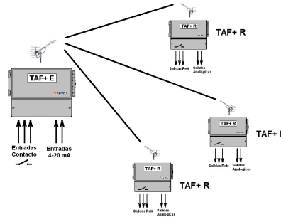
a) TAF E + n x TAF R
